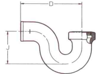
TAP P-TRAP
